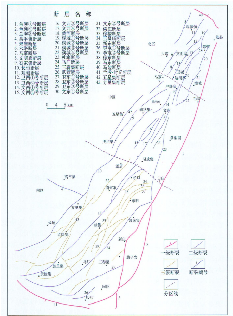
图1 东濮凹陷断裂系统 Fig. 1 Fault systems in Dongpu Sag
