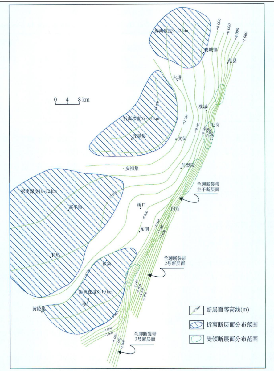
图 5 兰聊断层主断层面及深层拆离断层面构造等高线 Fig. 5 Structural contour of the major fault plane and the deep detachment fault plane of the Lanliao fault (兰聊断裂带主干断层面指控制古近系沉积的盆地东部边缘断层面,其中,断层面 \leq 8\,000\text{ m} 的部分等高线为根据地震剖面解释得到的数据,断层面 > 8\,000\text{ m} 的等高线是根据剖面线层变形特征而推测的,并根据剖面面积和伸展量按平衡剖面原理计算拆离断层面深度。)
